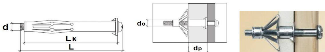
Метален дюбел за преградни стени - MOL
