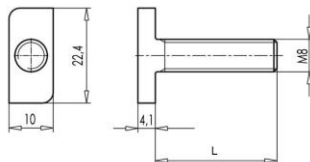
Т-болт М8, неръждаема стомана А2-70
