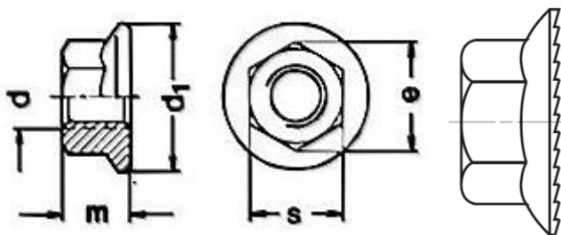
Гайка фланцова, DIN 6923, с накатка, неръждаема стомана A2-70
