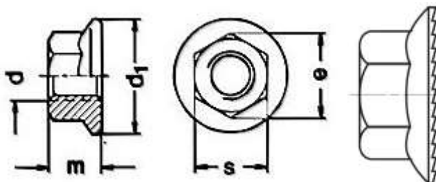
Гайка фланцова, DIN 6923, с накатка, поцинкована, клас на якост 6
