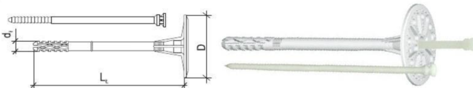
Дюбел за изолация с пластмасов пирон LTX
