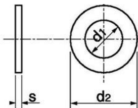
Шайба, подложна, DIN 125A, твърдост HV 200, без покритие
