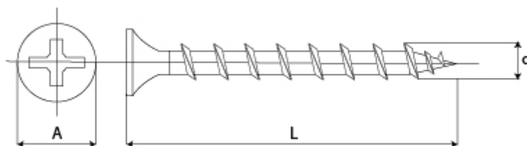
Винт за PVC с ЕДРА стъпка, PH, Zn
