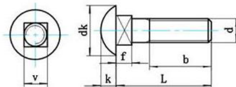
Carriage Bolt DIN 603, A2-70
