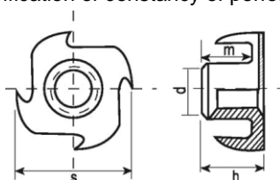
Drive-in Nut DIN 1624, Zn (6)
