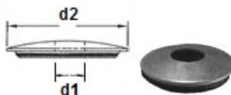
EPDM Washer
