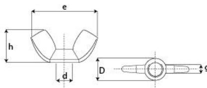
Wing Nut DIN 315A, Zn (6)
